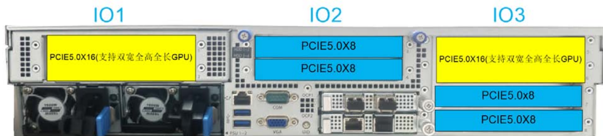
图 3-12 6 个 PCIe 插槽
