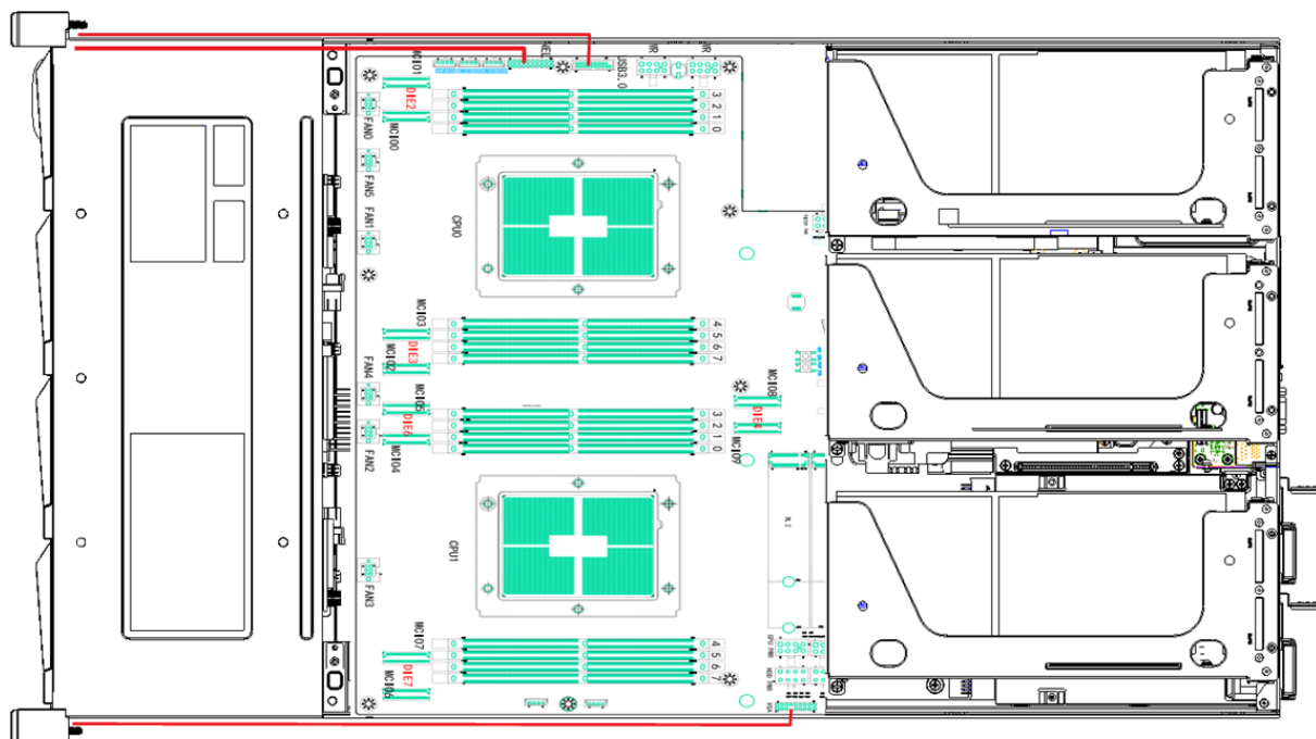
图 4-12 挂耳布线
