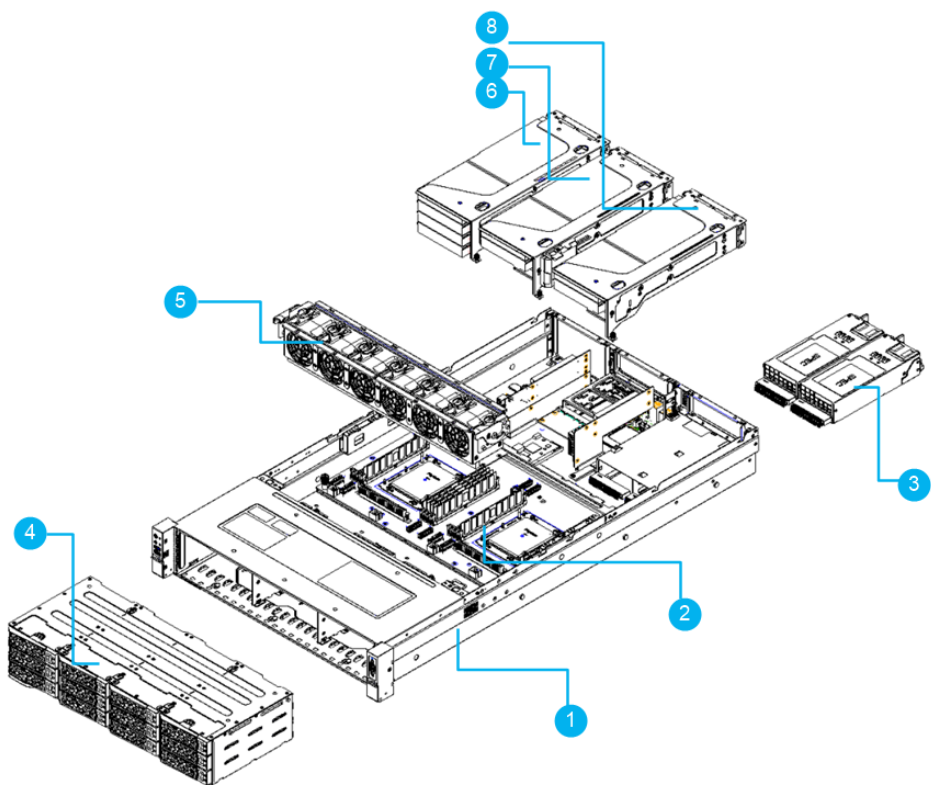
图 3-1 结构组成
