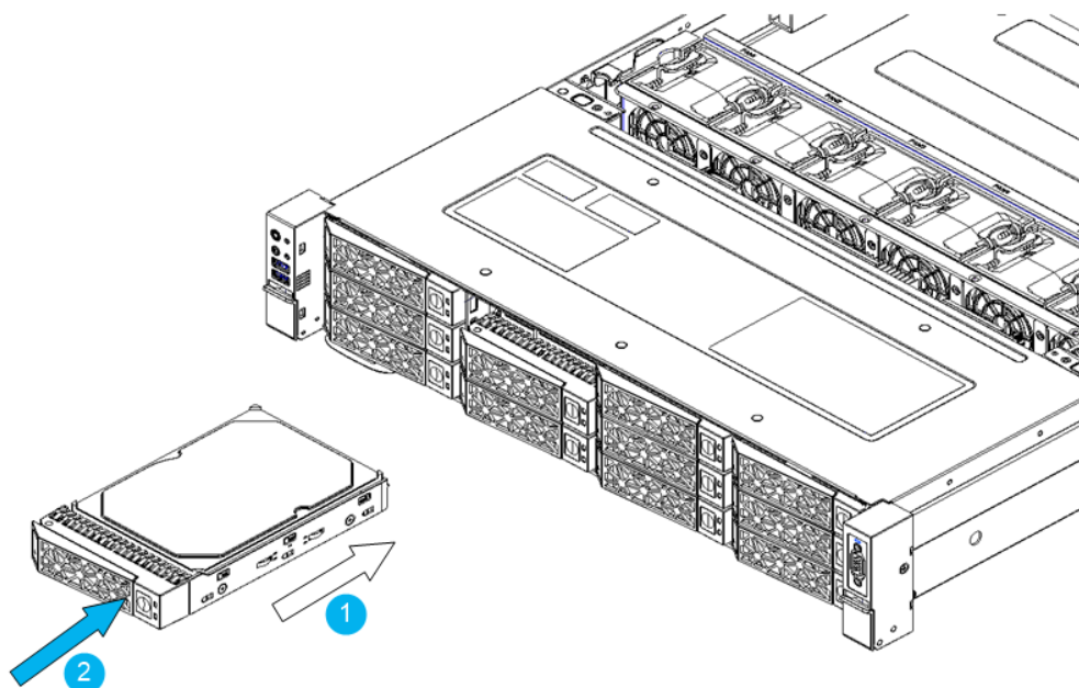
图 4-10 锁定硬盘
