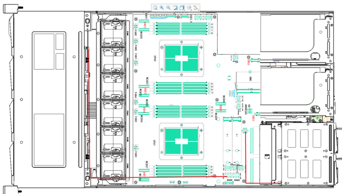
图 4-11 电源布线
