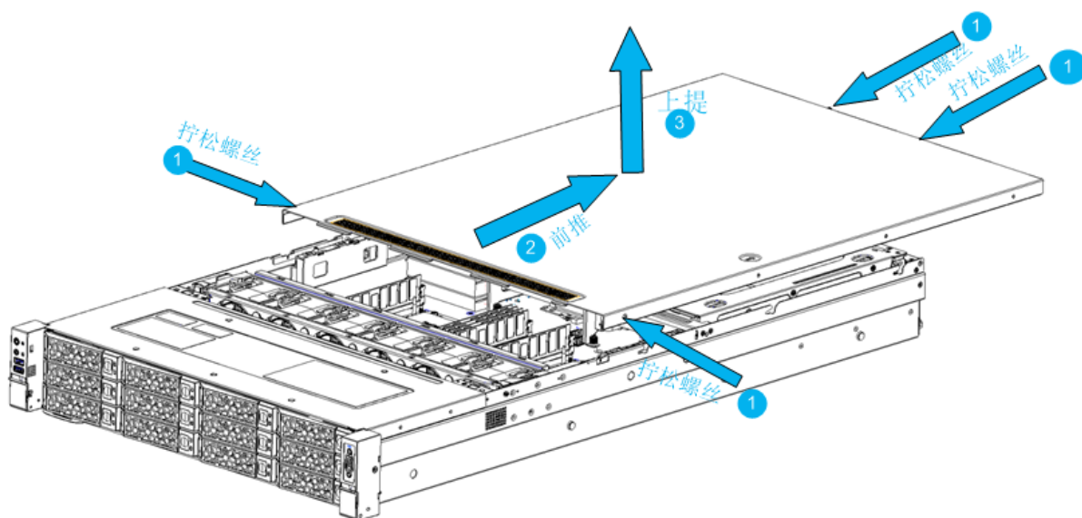
图 4-5 上盖开启
