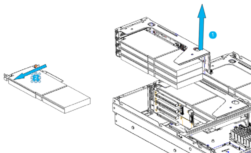
图 4-20 PCIe 卡拆卸
