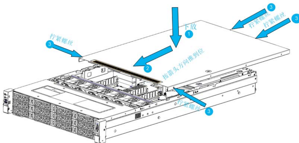
图 4-6 上盖闭合
