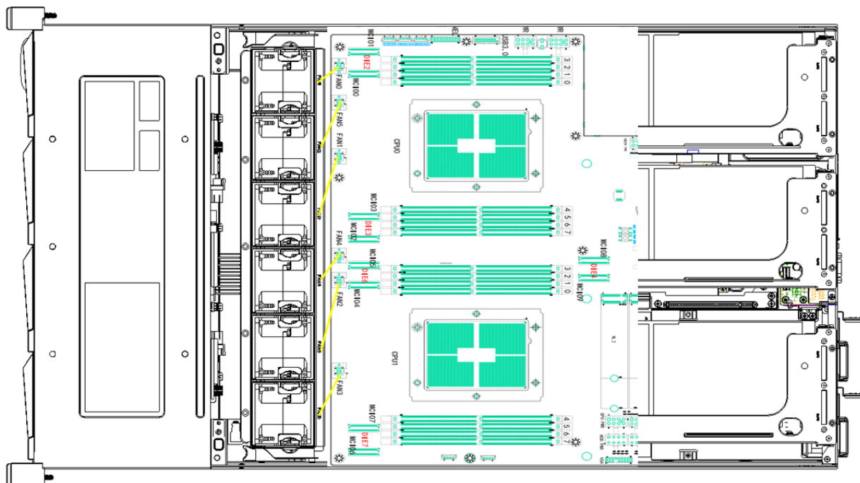
图 4-24 风扇布线
