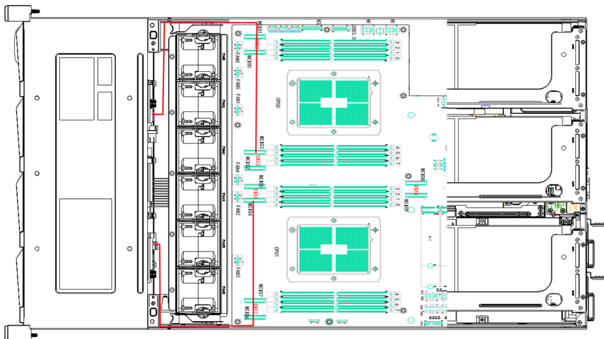
图 4-26 NVME 硬盘布线
